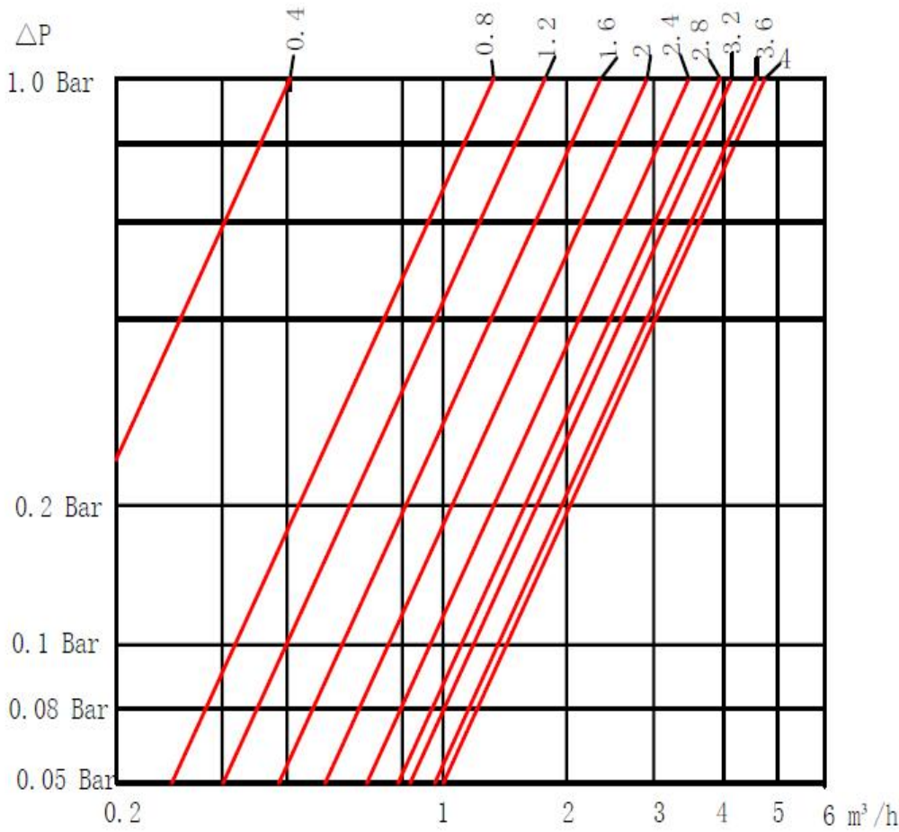
压力降与流量曲线：DN20
