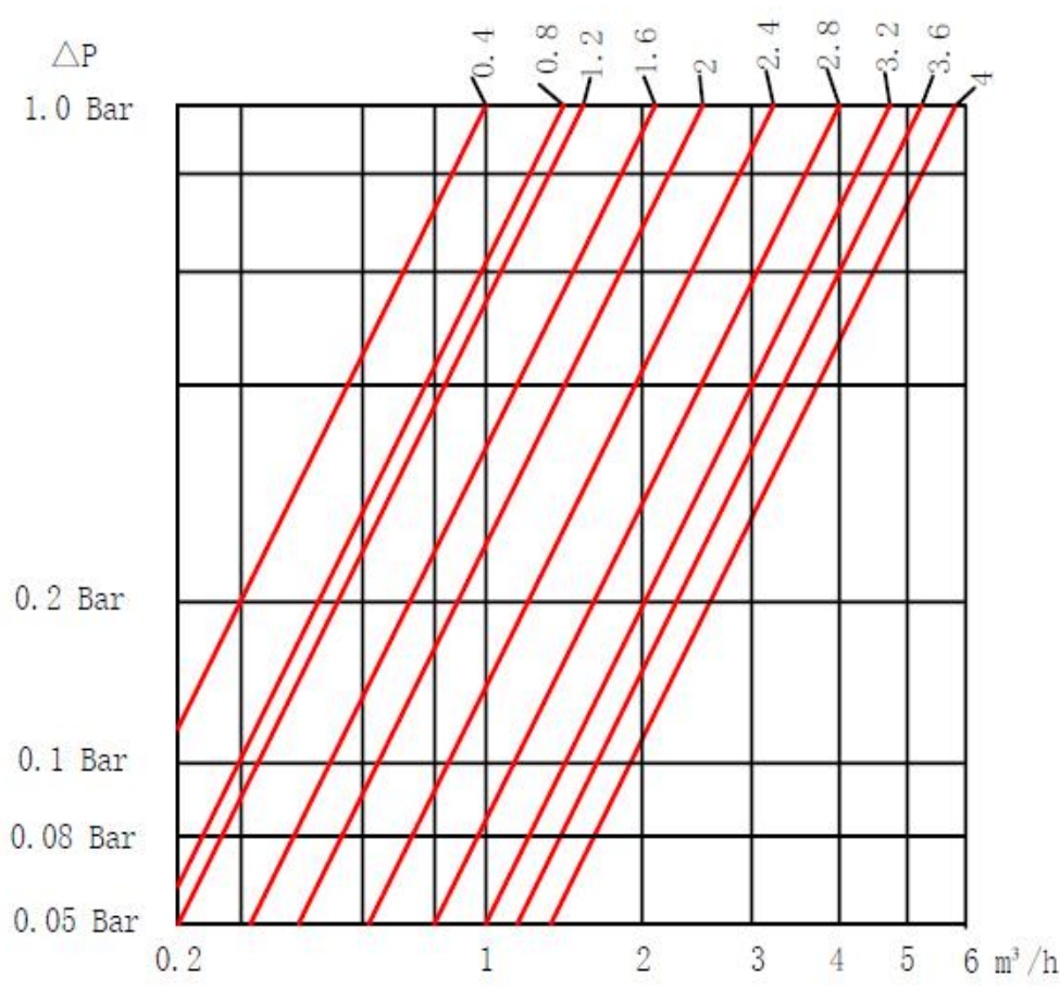
压力降与流量曲线：DN32
