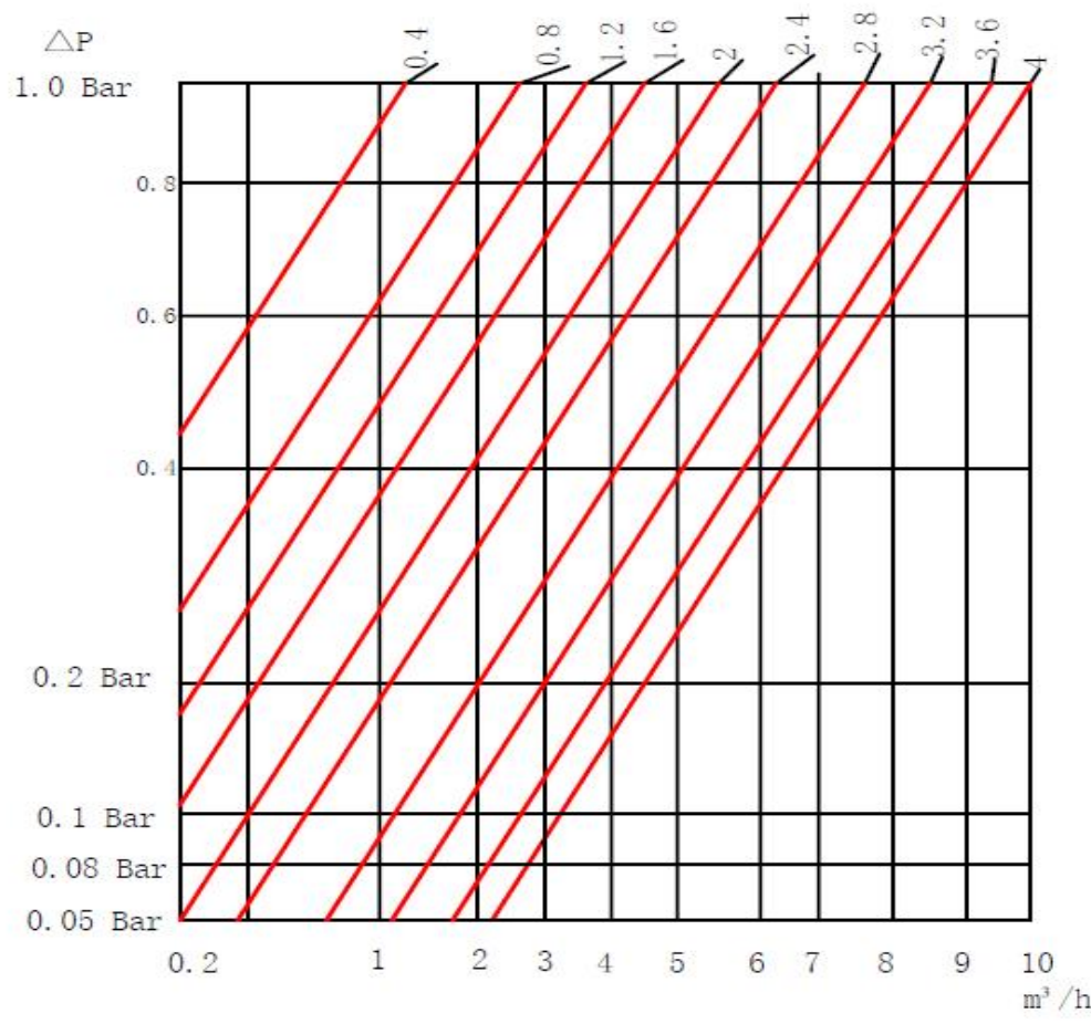
压力降与流量曲线：DN40
