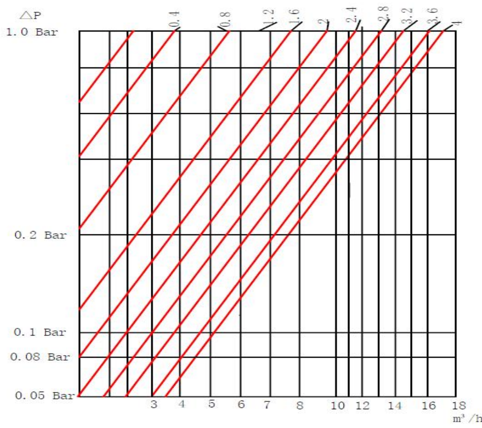
压力降与流量曲线：DN50
