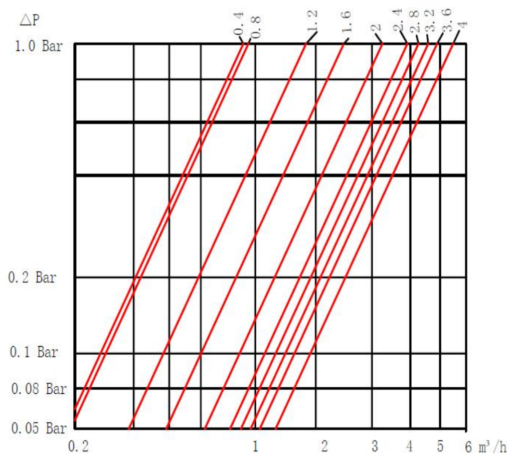
压力降与流量曲线：DN25
