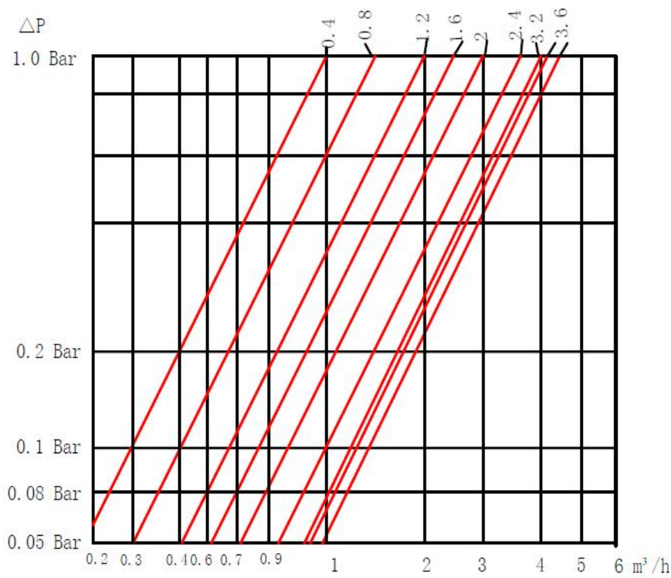
压力降与流量曲线：DN15
