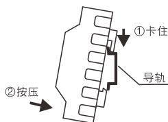
安装图
