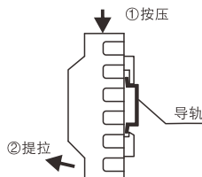
拆卸图
